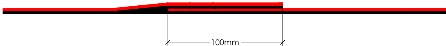
1 Roll End Detail Scale: 1:2
